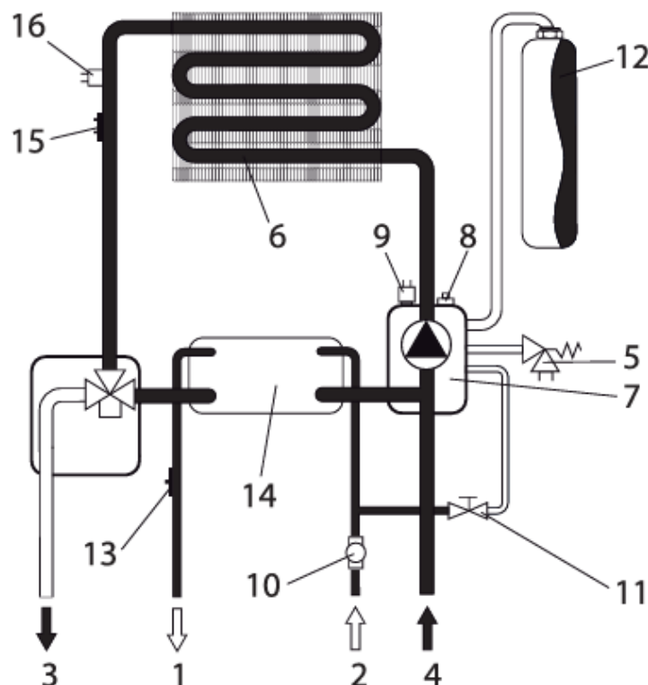
Гидравлическая схема в режиме ГВС
